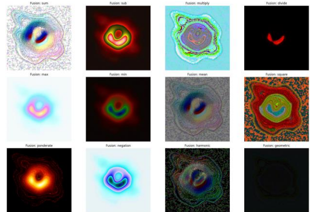
Fig. 17. Interference patterns for M87 EHT
