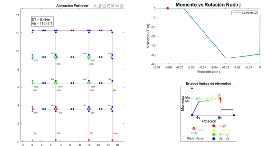
Fig 17. Secuencia de daño en los elementos estructurales.
