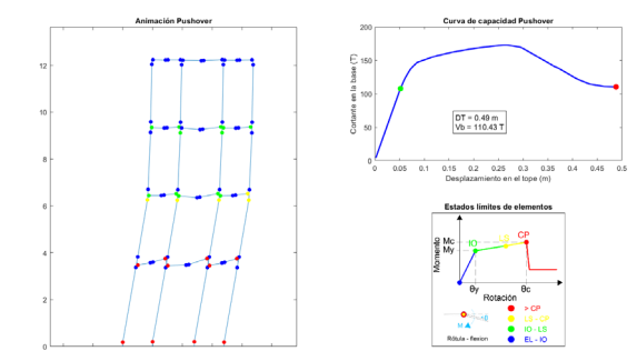
Fig 18. Animación del análisis Pushover.
