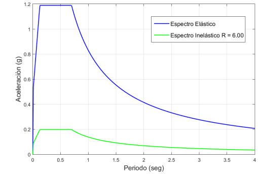
Fig 9. Espectro de diseño [20].
