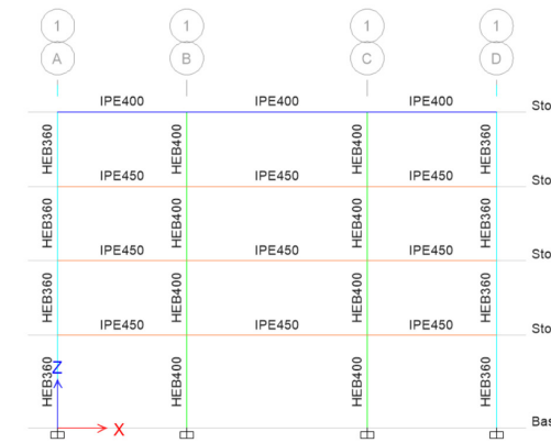
Fig 8. Pórtico en análisis [20].
