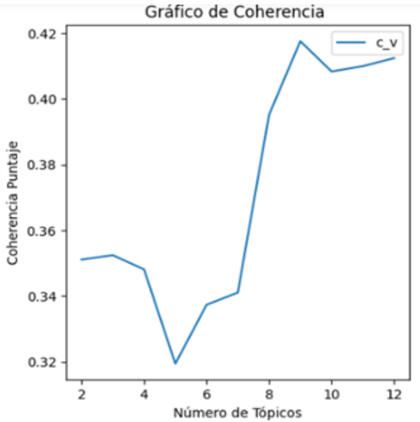
Fig. 3. Métrica de coherencia
